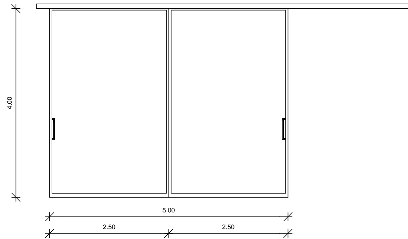
DRSNA VRATA V1 svetla odprtina: 4,0 x 5,0 m
