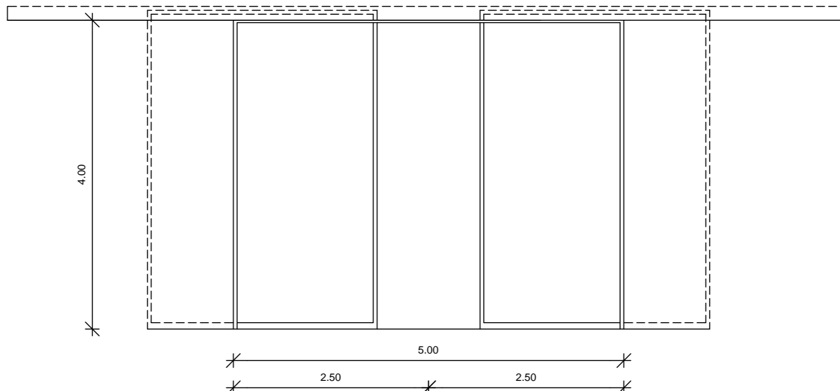
DRSNA VRATA V2 svetla odprtina: 4,0 x 5,0 m
