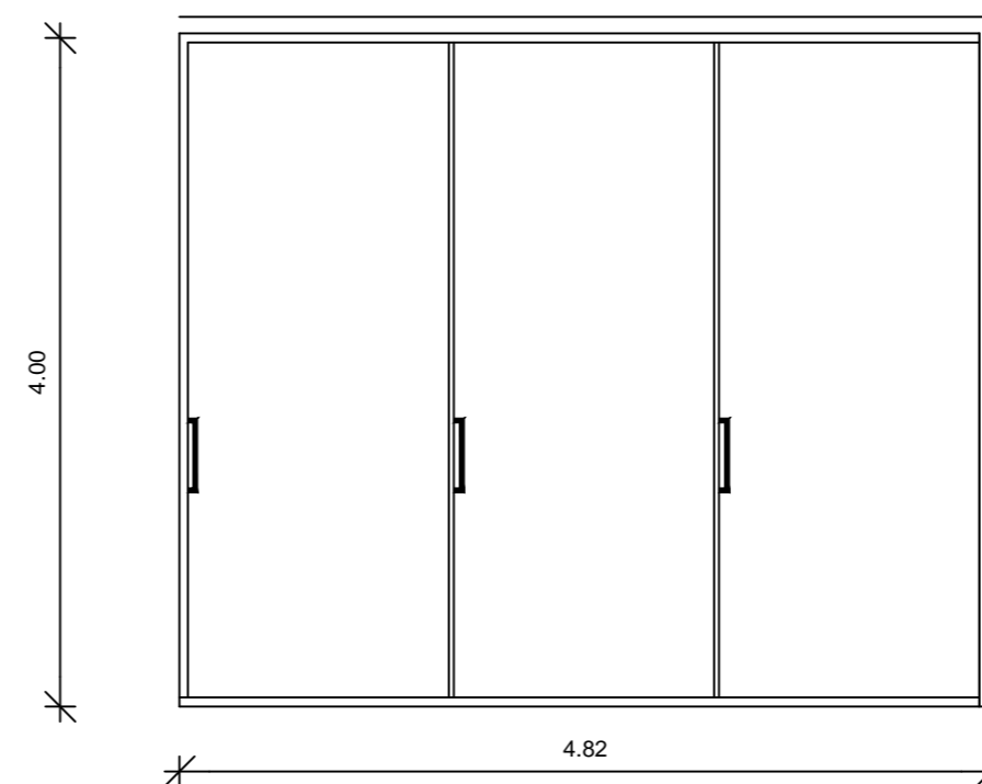
DRSNA VRATA V3 svetla odprtina: 4,0 x 4,82 m
