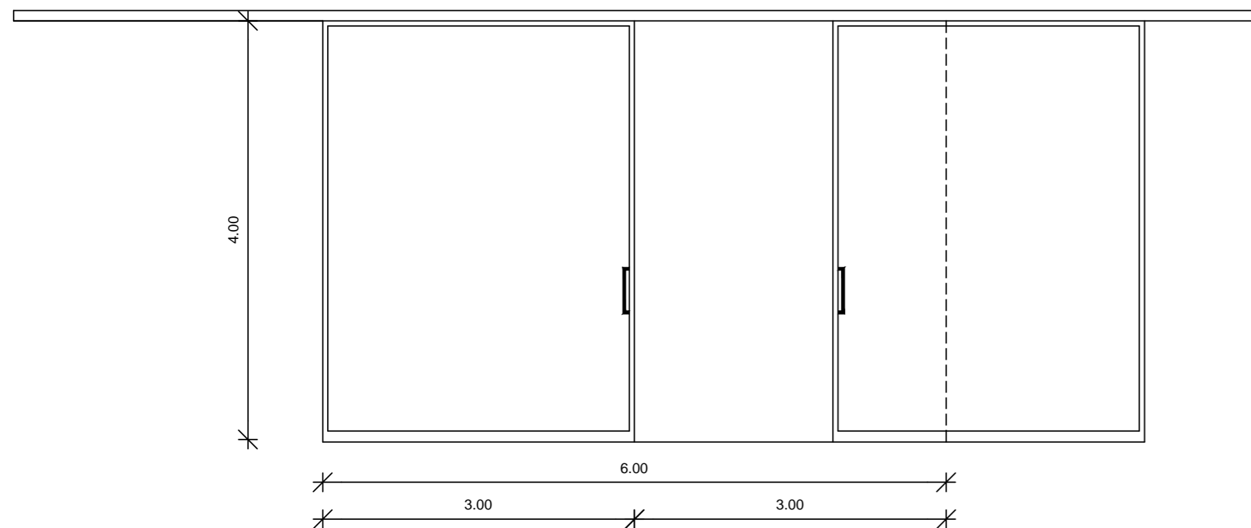
DRSNA VRATA V3 svetla odprtina: 4,0 x 6,0 m
